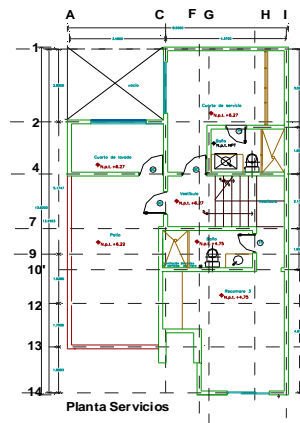
Planta Servicios
