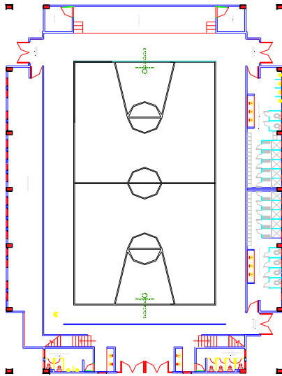
PLANTA BAJA
